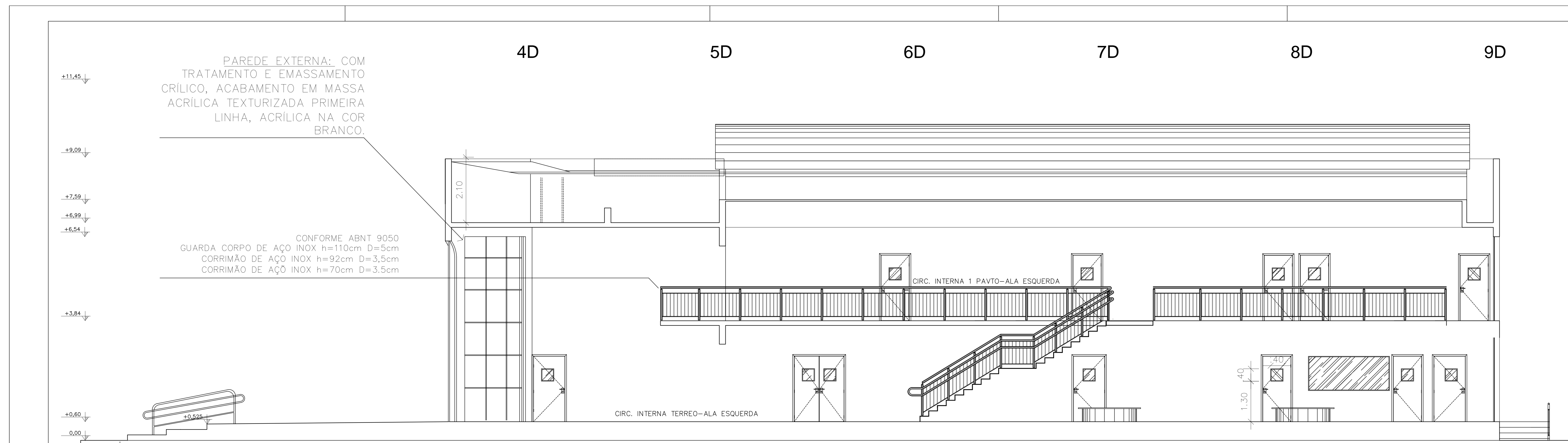
CORTE D-D ESCALA: 1/50
