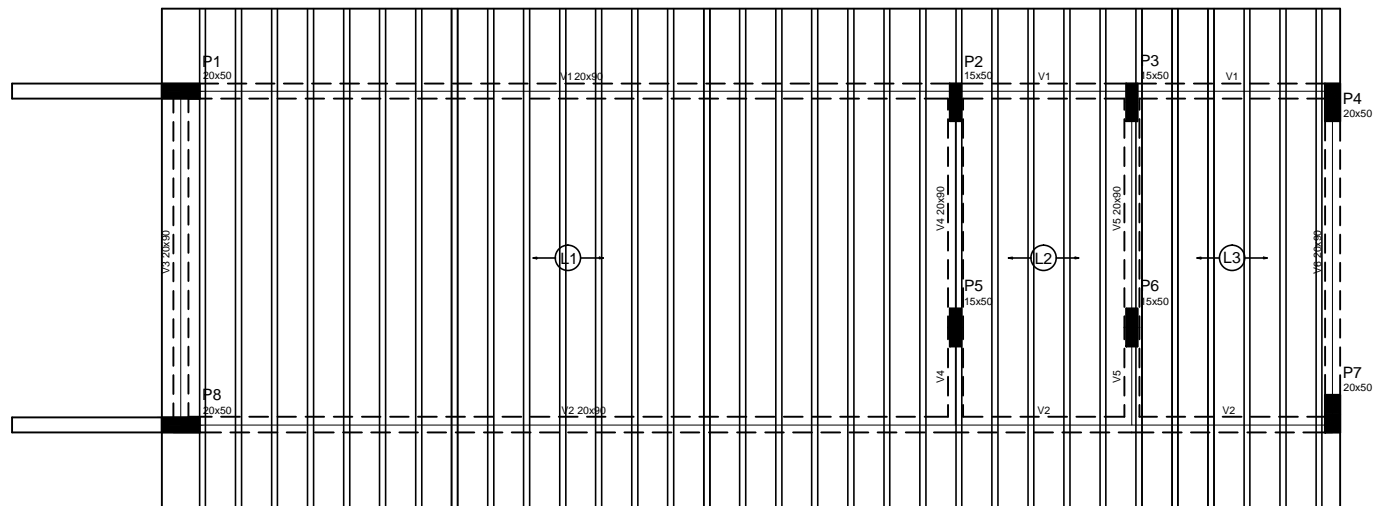
Forma do pavimento 1 PAV escala 1:50
