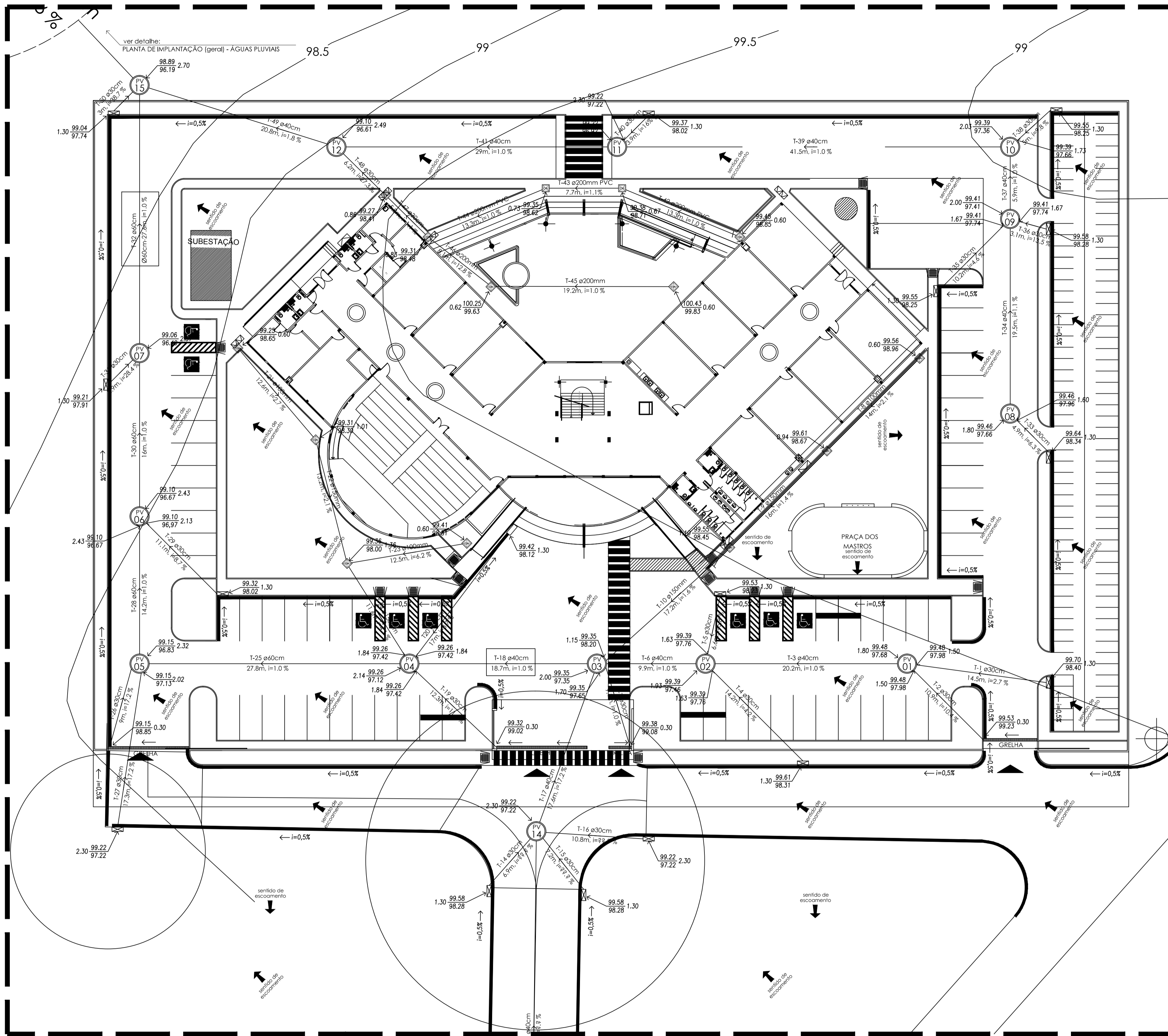
01 PLANTA DE IMPLANTAÇÃO (parcial) - ÁGUAS PLUVIAIS ESCALA 1 : 250
