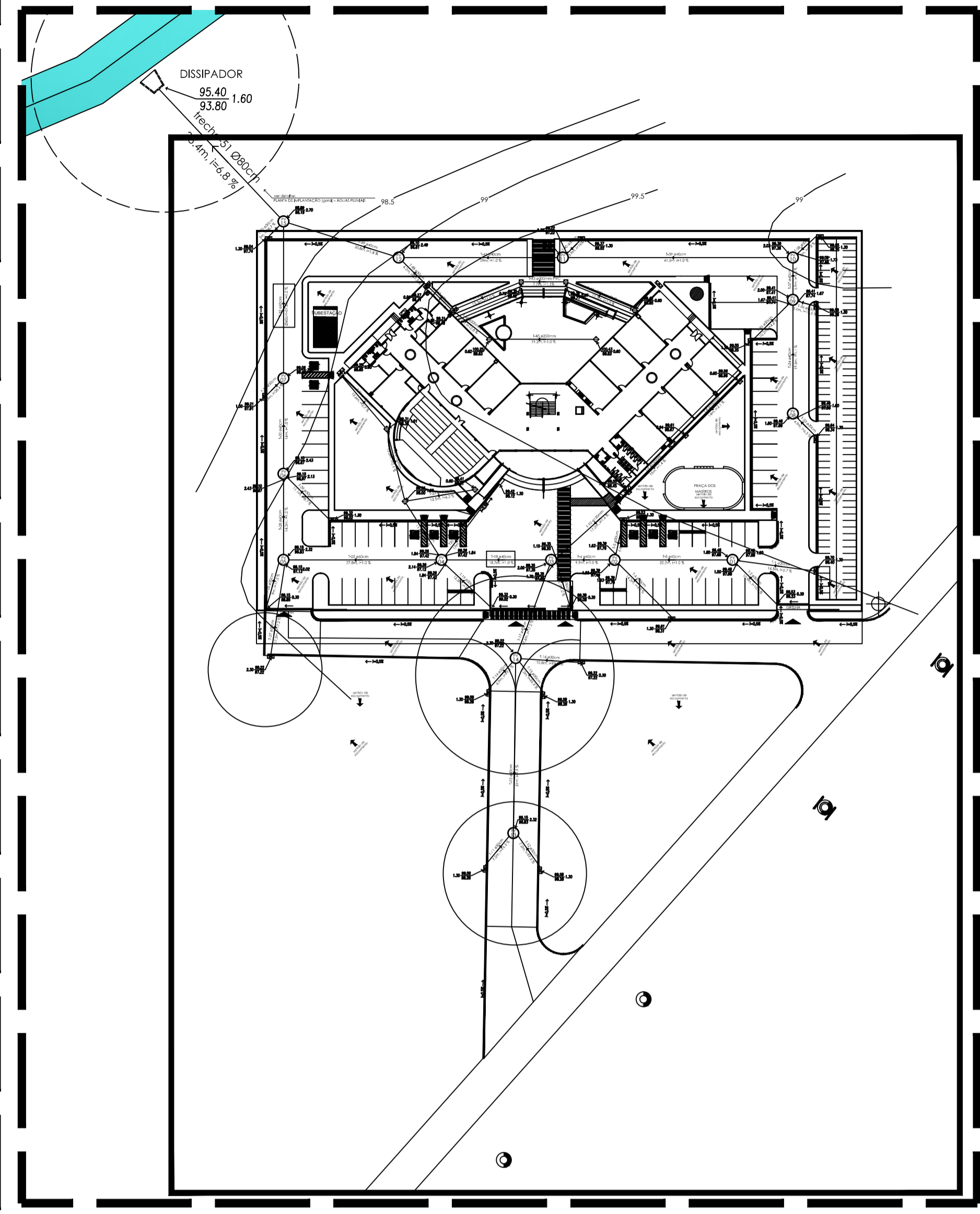
02 PLANTA DE IMPLANTAÇÃO (geral) - ÁGUAS PLUVIAIS ESCALA 1 : 750
