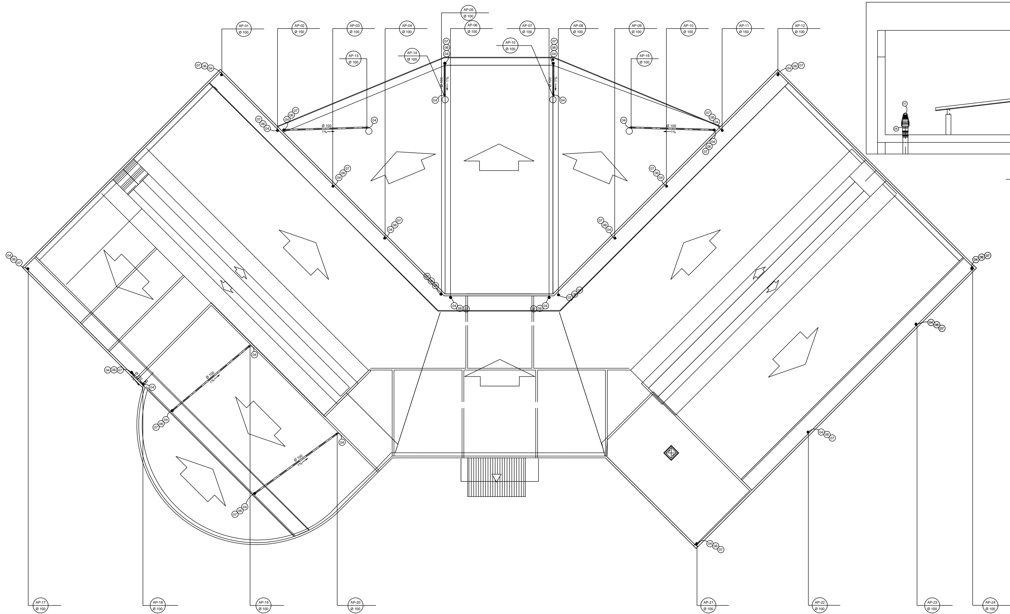
ESQUEMA GERAL - COBERTURA ESCALA 1 : 100
