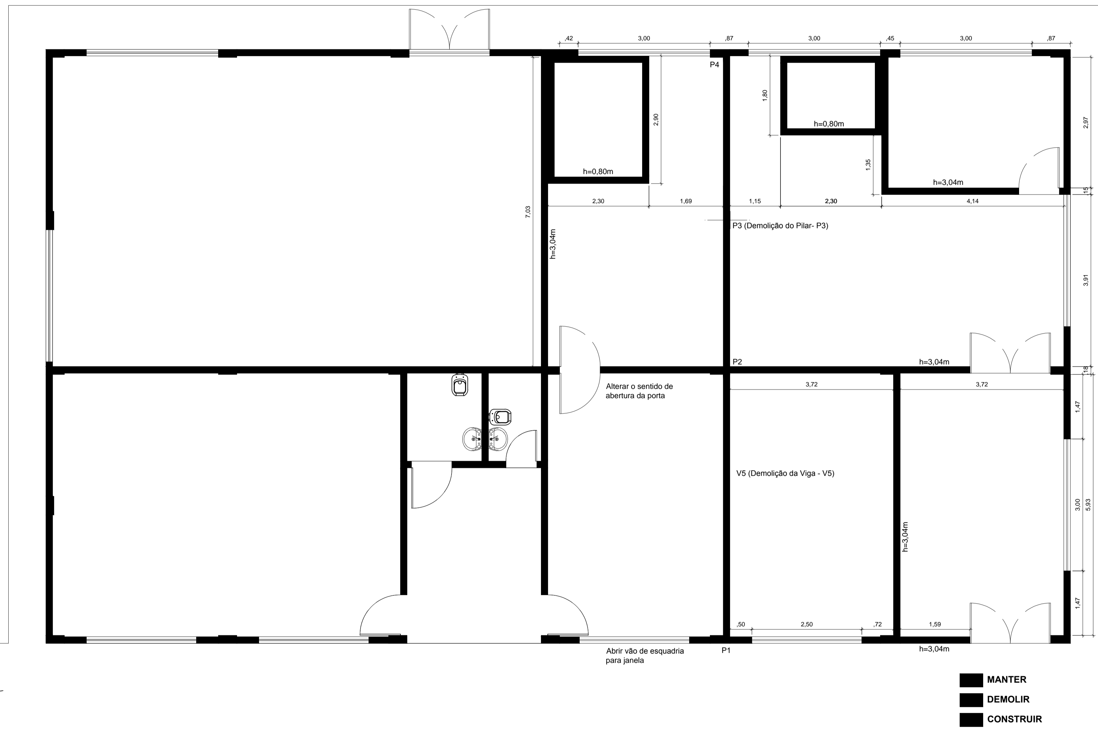
PLANTA DE REFORMA ESCALA 1/50
