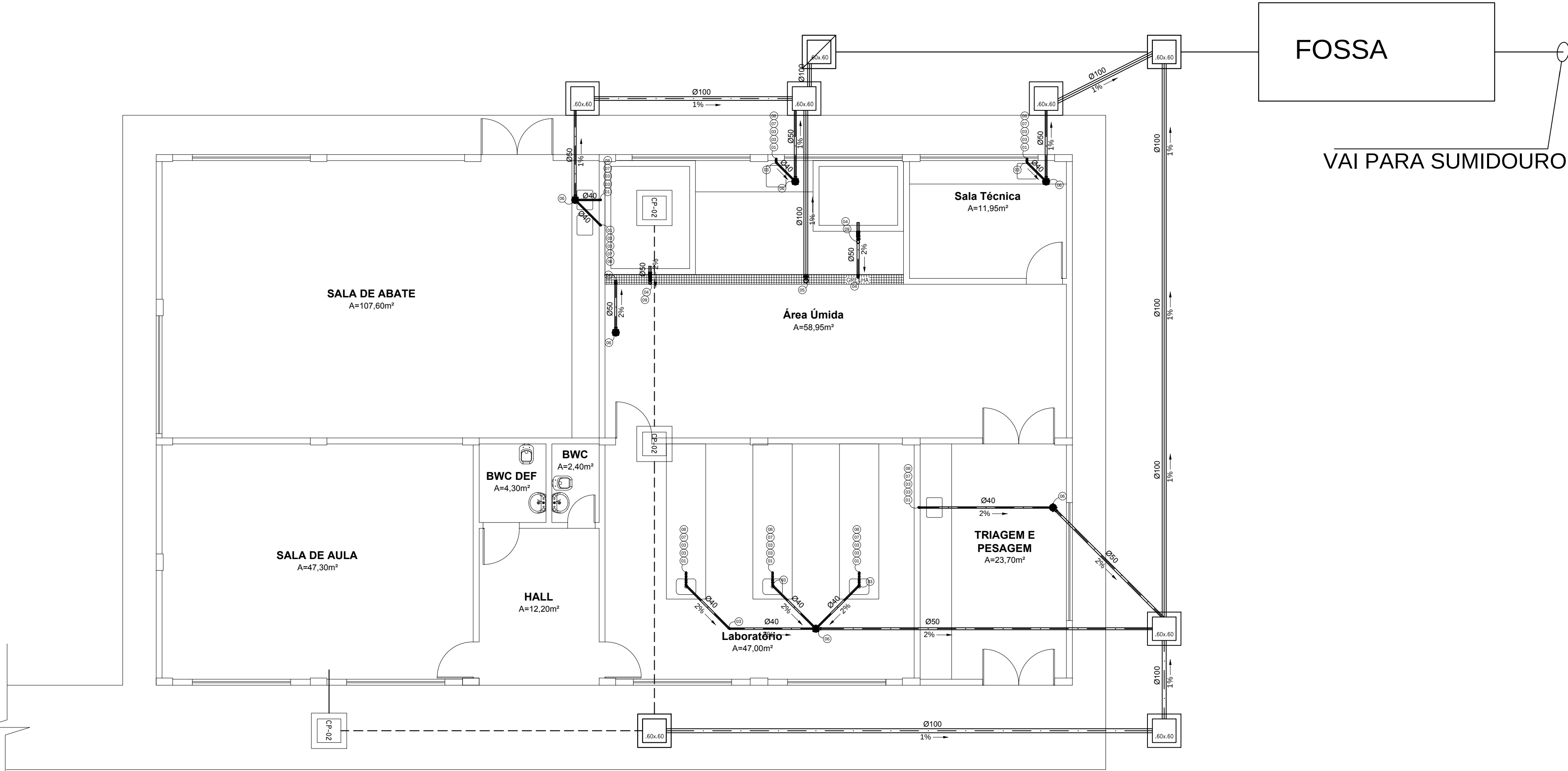
INSTALAÇÕES DE ESGOTO SANITÁRIO ESCALA: 1:75
